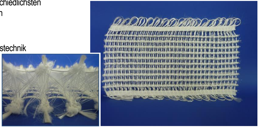
Abstandsgewirke mit AR-Glasfasern in den Deckflächen Spacer fabric with AR glass fibres in the cover faces
